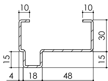
Huisserie T5
