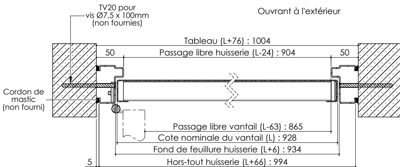
Huisserie T5
