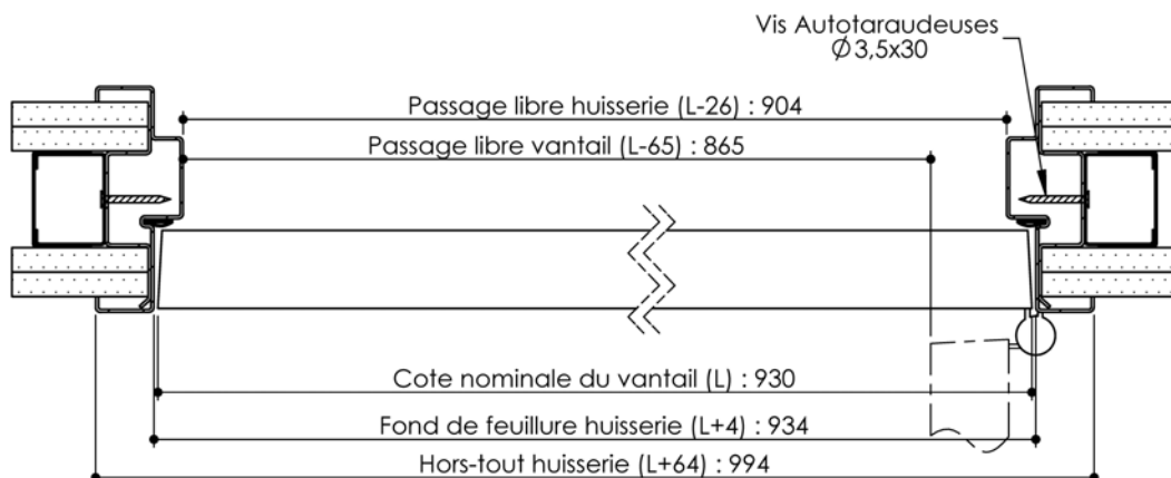
Seuil à la suisse + joint balai
